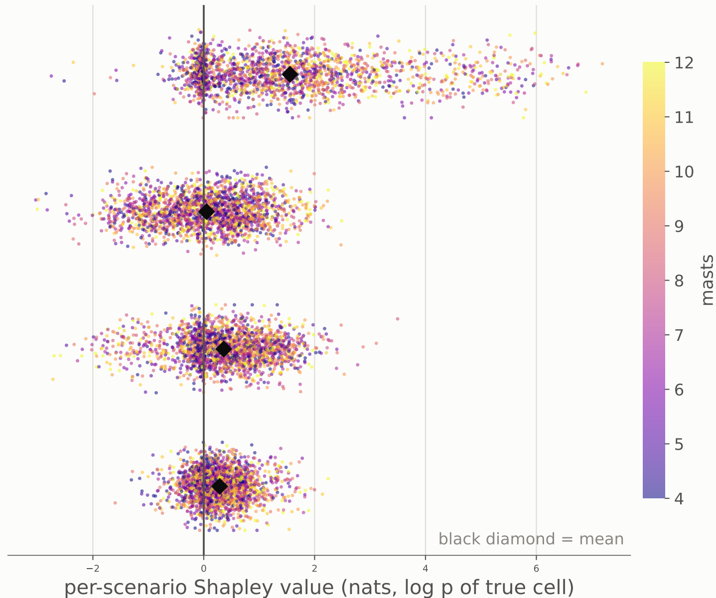
B. Per-scenario values — DeepSets
